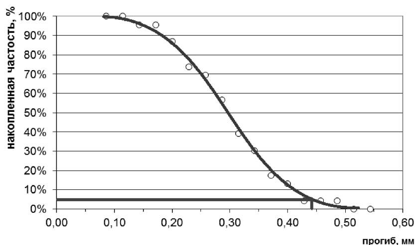
Рисунок 2 – Определение фактического прогиба дорожной одежды для характерного участка с коэффициентом надежности 0,95
