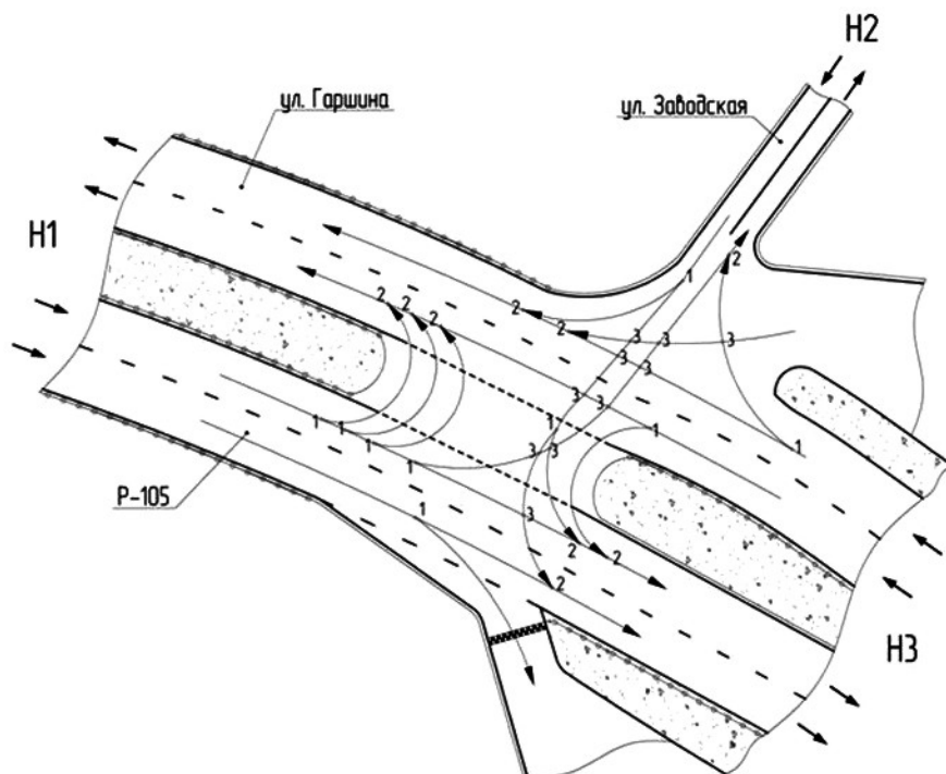
Рисунок 2 – Общее расположение конфликтных точек при существующей схеме ОДД
