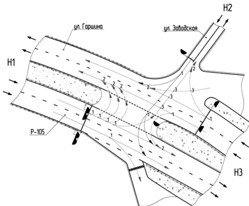
Рисунок 3 – Общее расположение конфликтных точек при предлагаемой схеме ОДД
