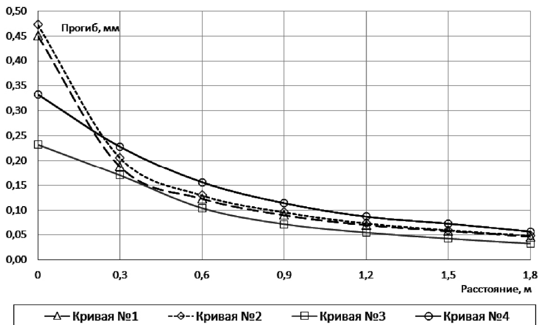
Рисунок 1 – Формы кривых чаши прогиба
