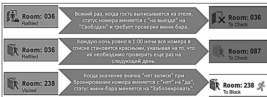
Рисунок 10 – Автоматический алгоритм действий изменения статуса мини-бара в номере
