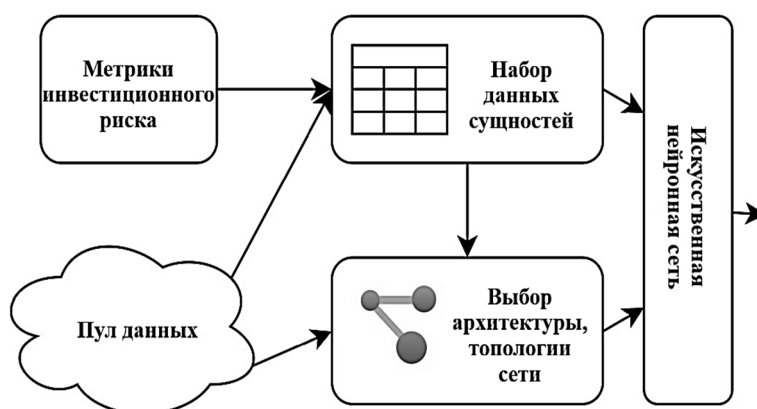
Рисунок 1 – Блок-схема использования нейронечеткого моделирования для оценки инвестиционных рисков (разработано автором)
