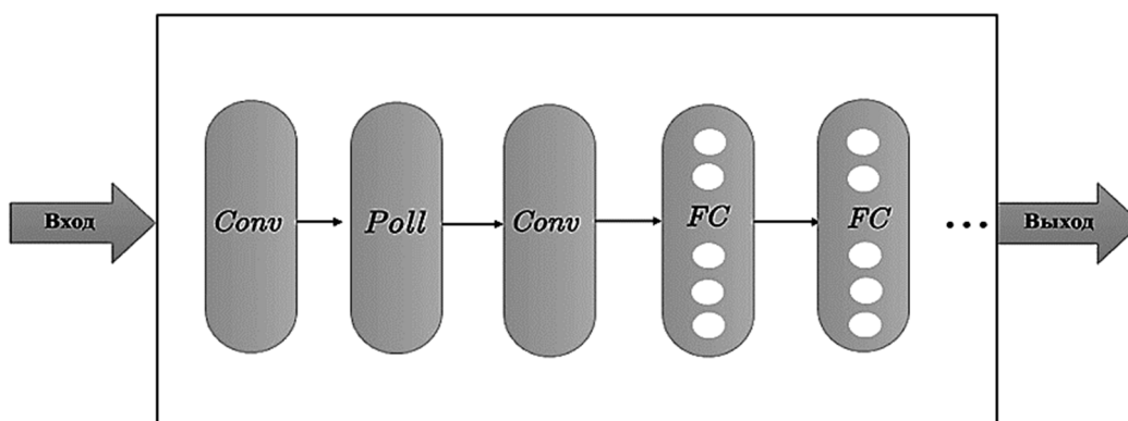
Рисунок 3 – Блок-схема одномерной CNN
