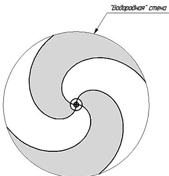
Рисунок 4 – Схематическое изображение однонаправленных движений солнечного ветра и водородной стены
