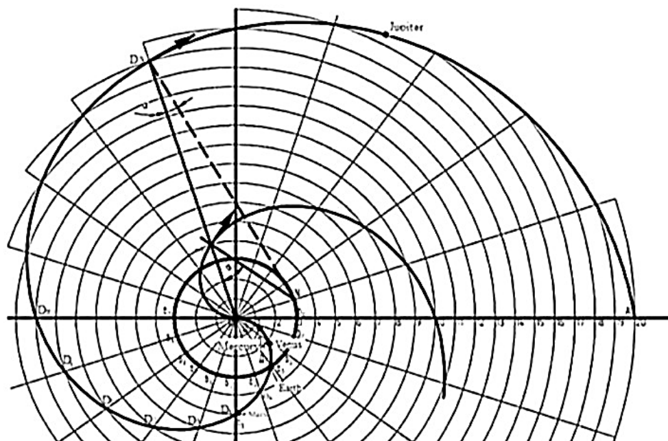
Рисунок 2 – Схематическое изображение движения солнечного ветра при повороте солнечной короны относительно ядра Солнца
